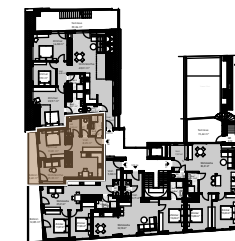
1. Dachgeschoss
